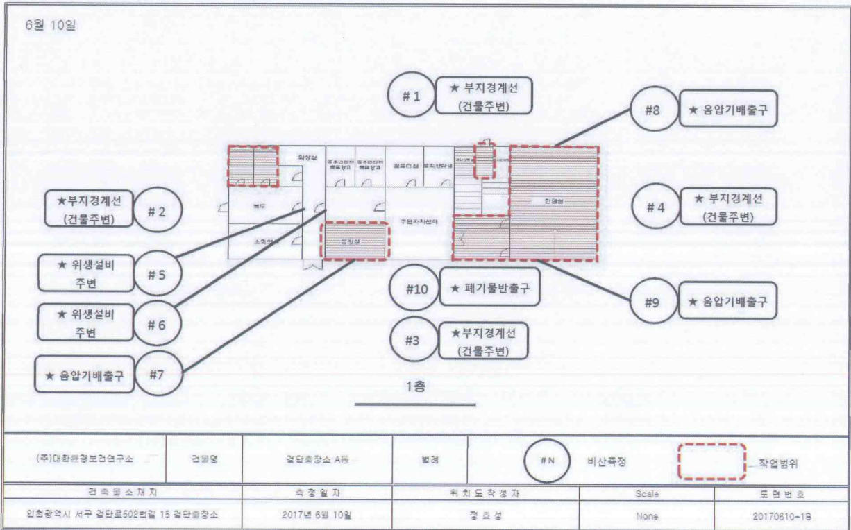
◆ 별첨2 - 비산측정지도 [ 검단출장소 청사 리모델링공사 석면폐기물 처리구역 ]
